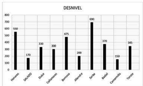
Gráfico 2: Desnivel de los ríos de la cuenca del Henares.
